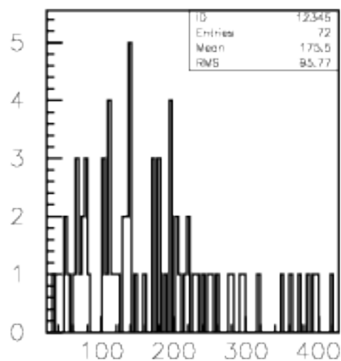
NEWQDC(:72)
