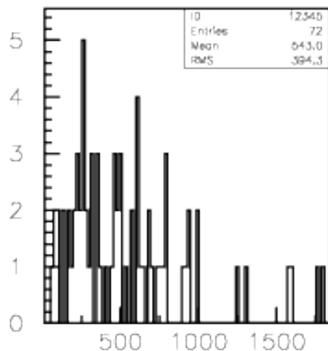
OLDQDC(:72)
